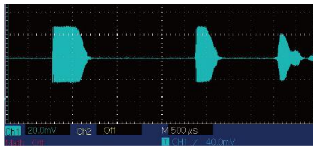
图 3：声压灵敏度
